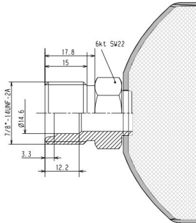
HANSA O-Ringe Anschluss 7/8"-14UNF HANSA O-ring connector 7/8-14UNF für Rohrgröße / tube size 16 mm / 5/8"
